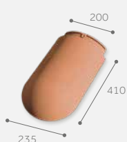
Final de limatesa universal
